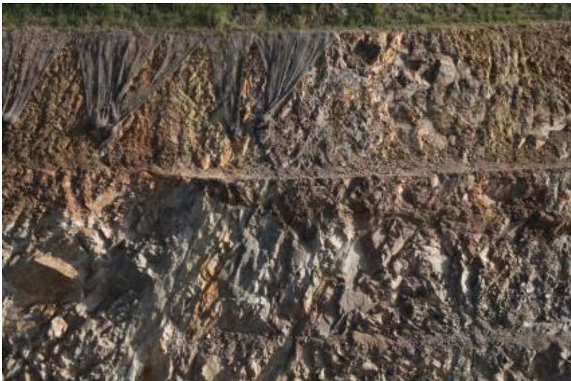
STA.4+840 중단부2
