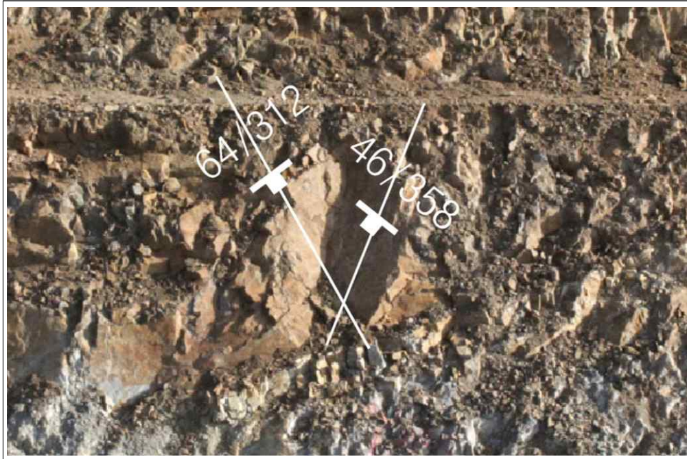
【그림 19】 C 영역에 발달한 불연속면
