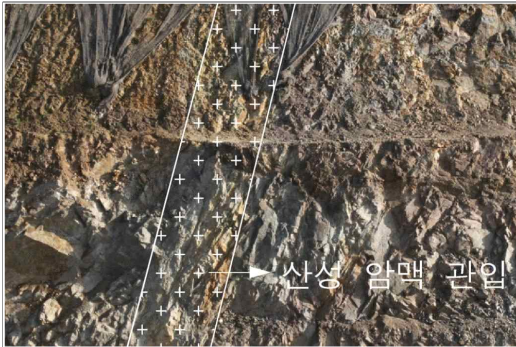
【그림 10】 A 영역 산성 암맥 관입
